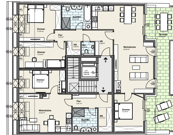
Dachgeschoss
